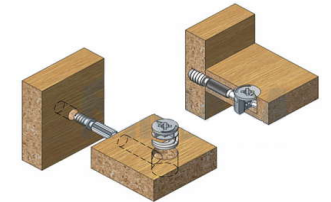
Эксцентриковая стяжка
