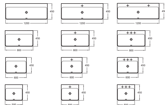
Раковины-чаши с отверстием для смесителя или без отверстий
